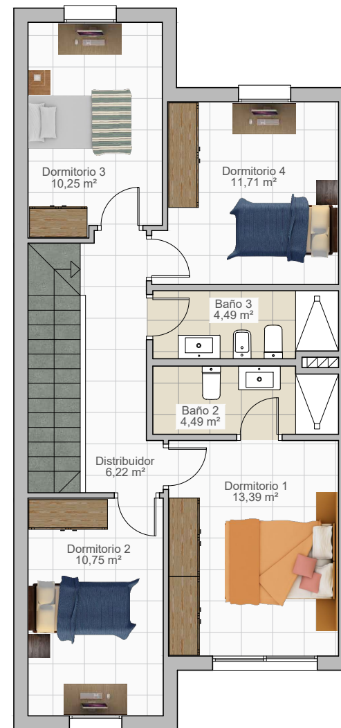
PLANTA PRIMERA
