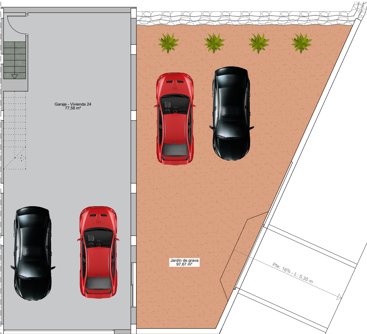
PLANTA SÓTANO
