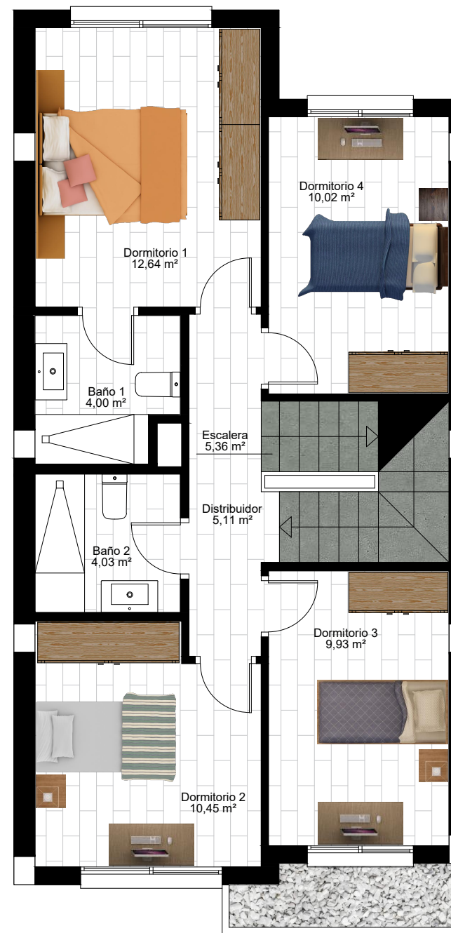
PLANTA PRIMERA
