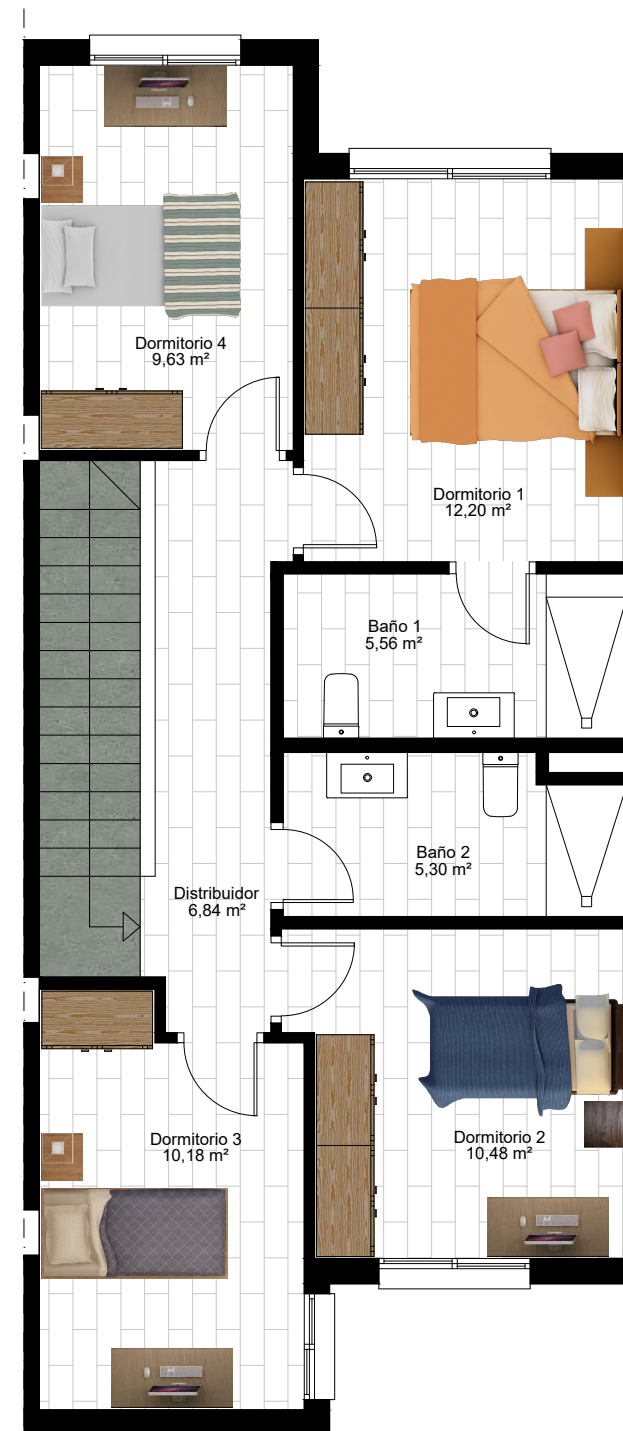
PLANTA PRIMERA
