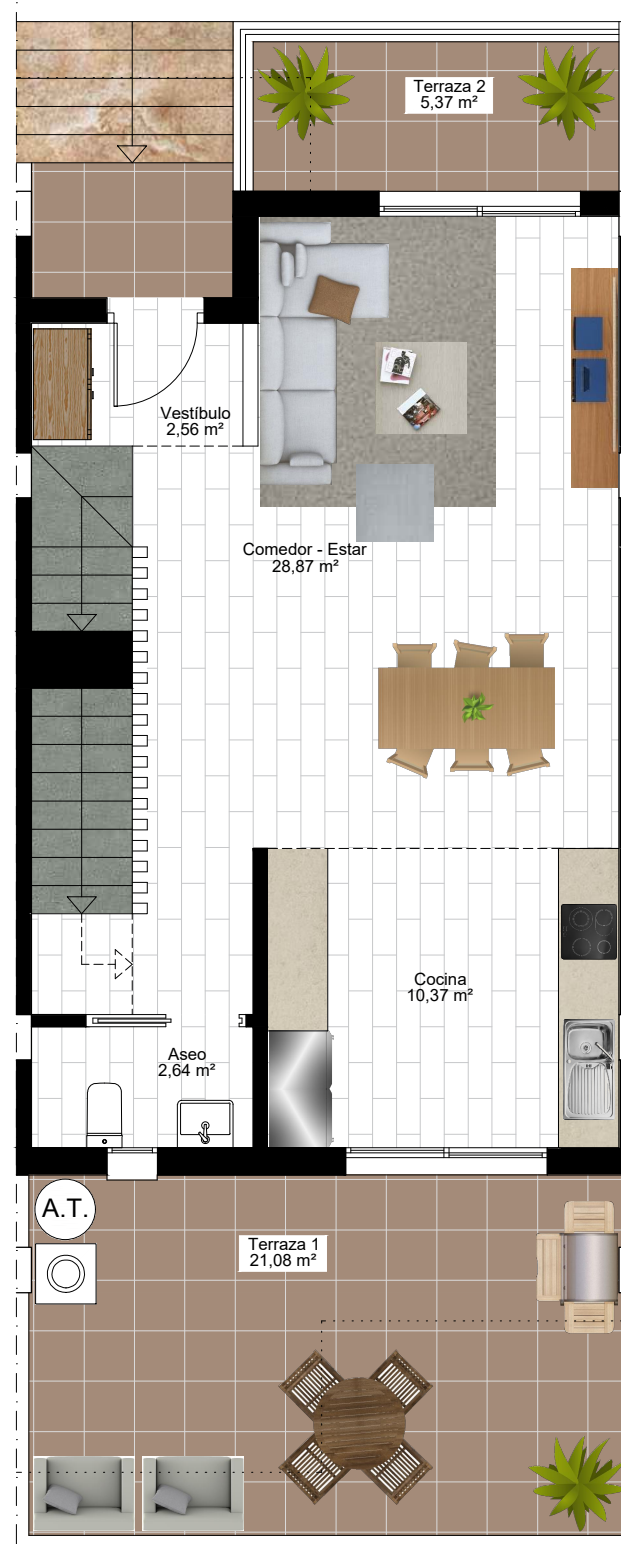
PLANTA BAJA
