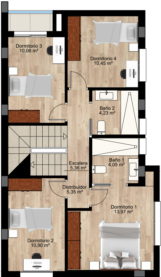
PLANTA PRIMERA
