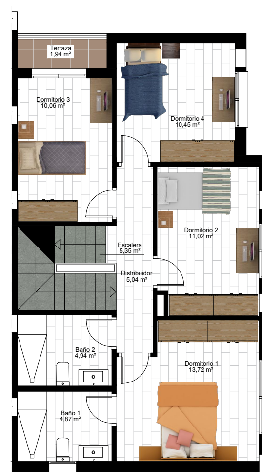
PLANTA PRIMERA
