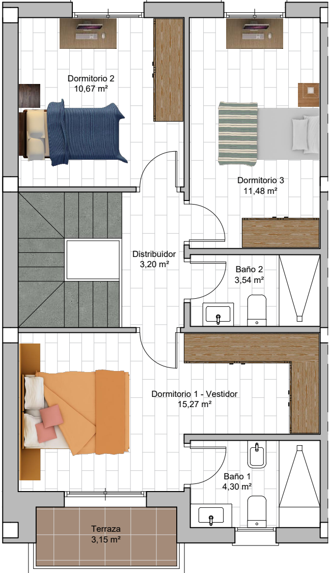
PLANTA PRIMERA
