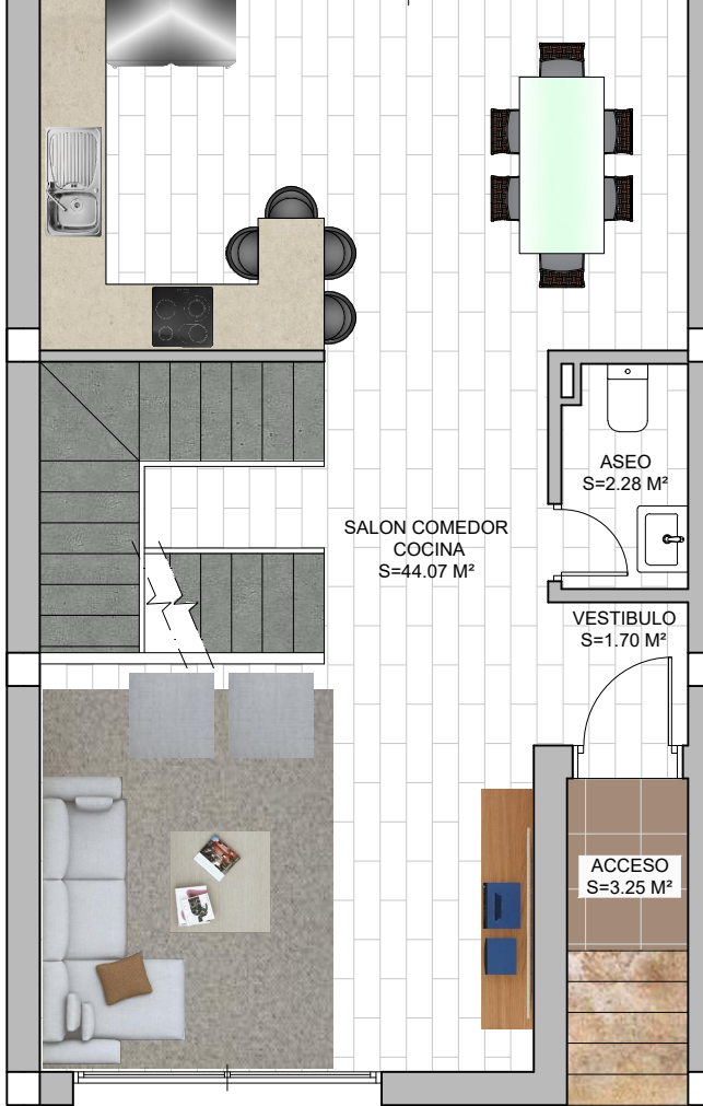
PLANTA BAJA
