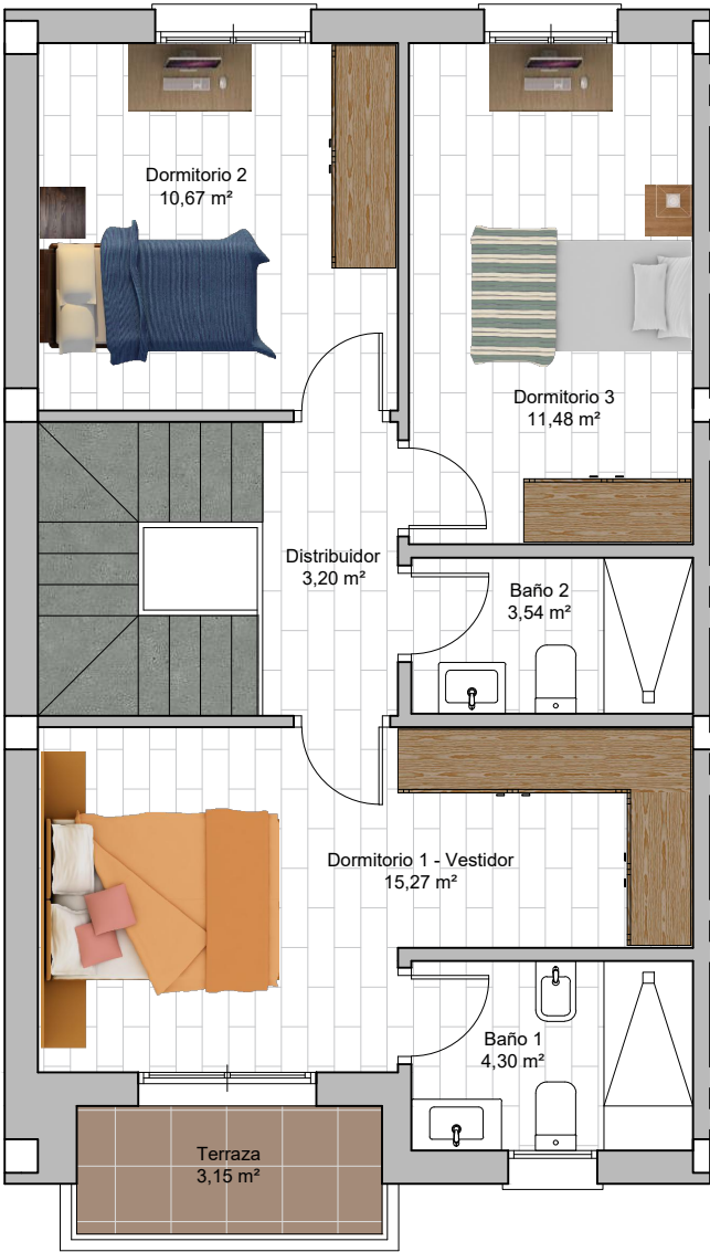
PLANTA PRIMERA
