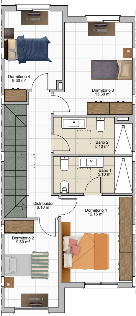
PLANTA PRIMERA
