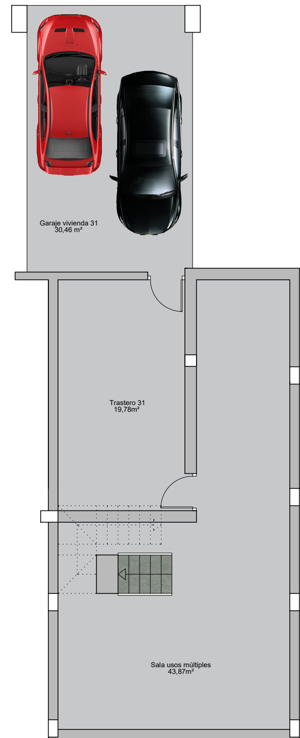
PLANTA SÓTANO
